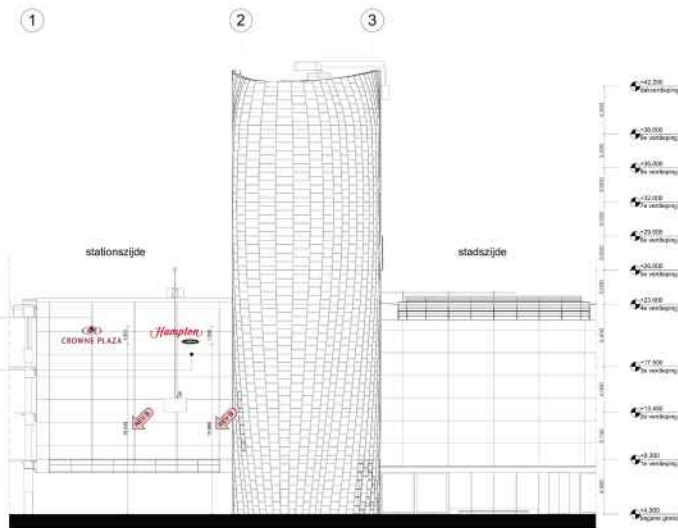
Zuidoostgevel (Kopgevel)
