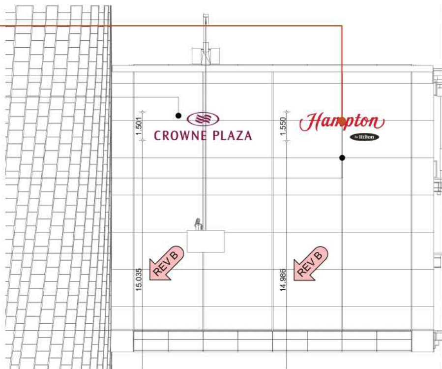
GEVELFRAGMENT 1:200
