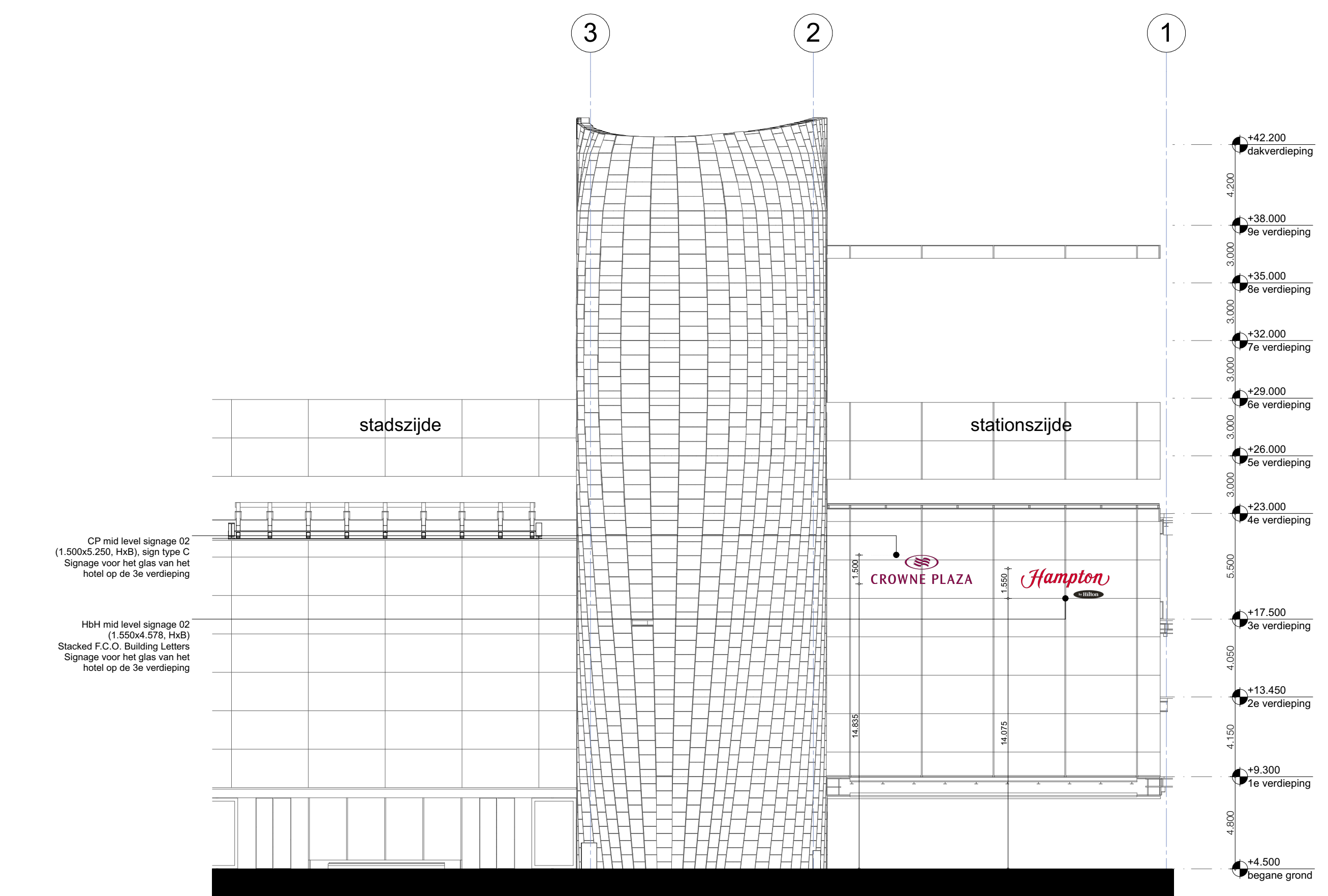
Zuidoostgevel (Kopgevel)
