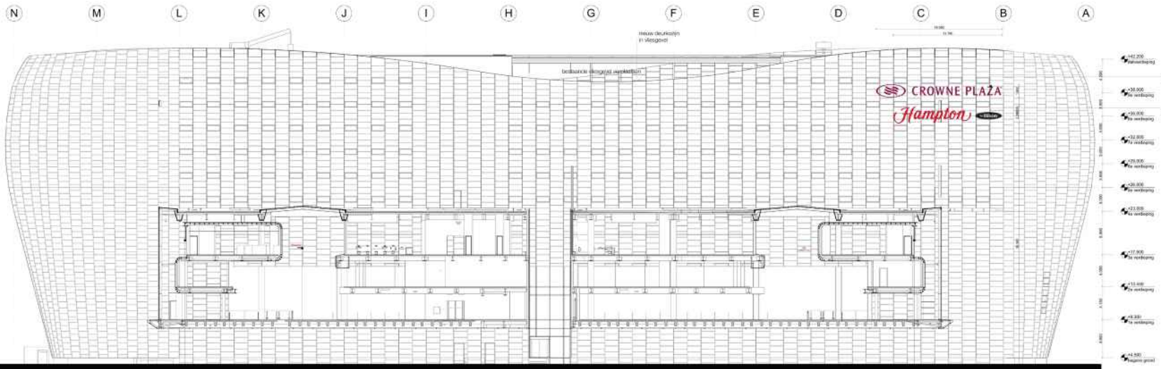
Zuidwestgevel (Langsgevel stationszijde)
