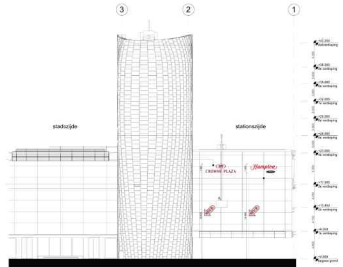
Noordwestgevel (Kopgevel)
