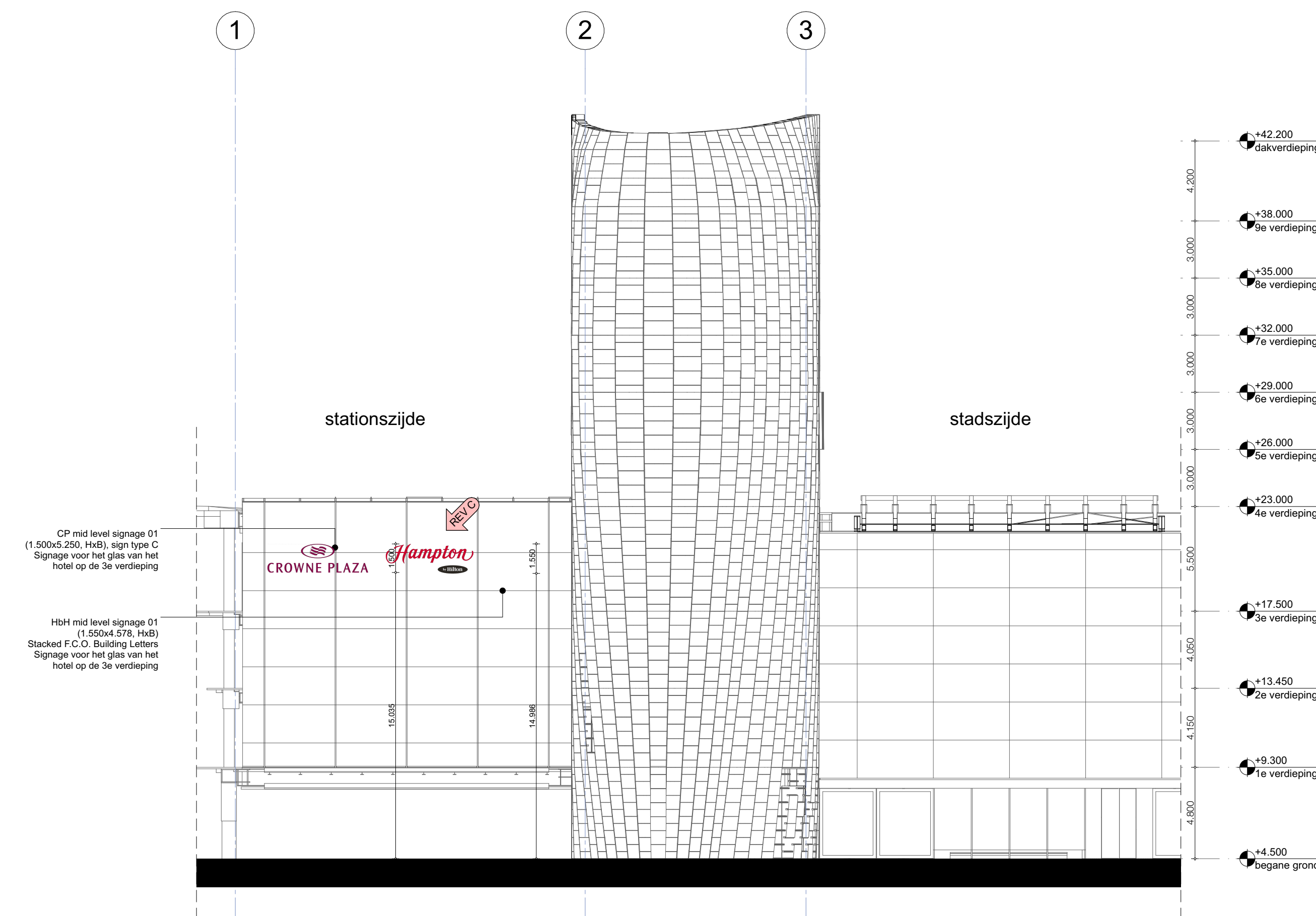
Zuidoostgevel (Kopgevel)
