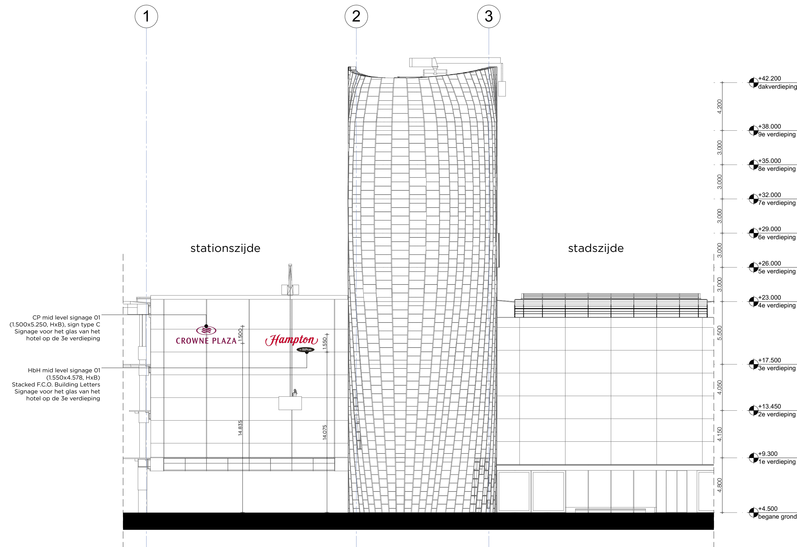
Zuidoostgevel (Kopgevel)
