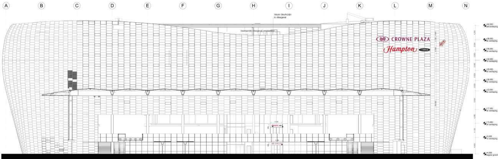
Noordoostgevel (Langsgevel stadszijde)
