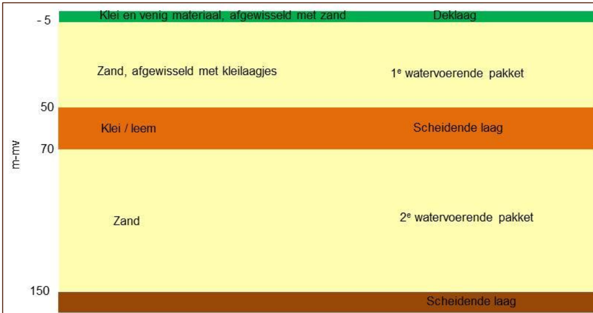
Figuur 3: Schematische weergave bodemopbouw ter plaatse van plangebied Merwedekanaalzone
