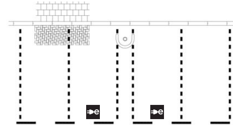
Opstellingsvoorbeeld 1: plaatsing laadpunt en tegel in parkeervak
