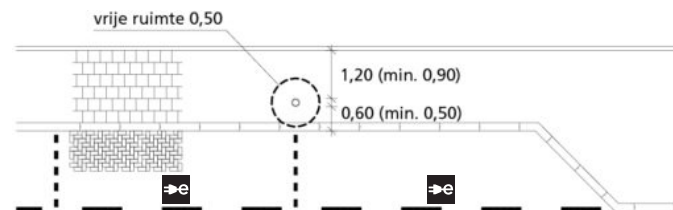
Opstellingsvoorbeeld 1: plaatsing tegel en laadpunt bij langsparkeervakken
