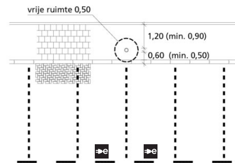
Opstellingsvoorbeeld 2: plaatsing laadpunt op trottoir en tegel in parkeervak
