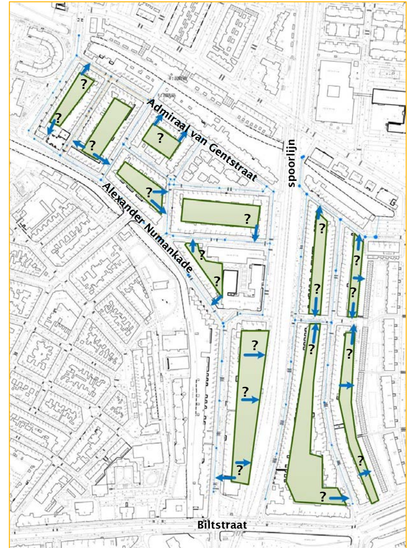
Inventarisatie van tuinen en openingen (pijlen) waar mogelijk een gezamenlijke regenpijp kan aansluiten op het nieuwe hemelwaterriool
