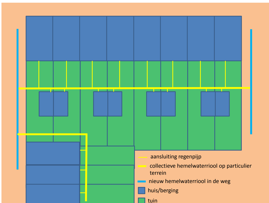
Een schetsmatige uitwerking van een collectieve afvoer door meerdere tuinen
