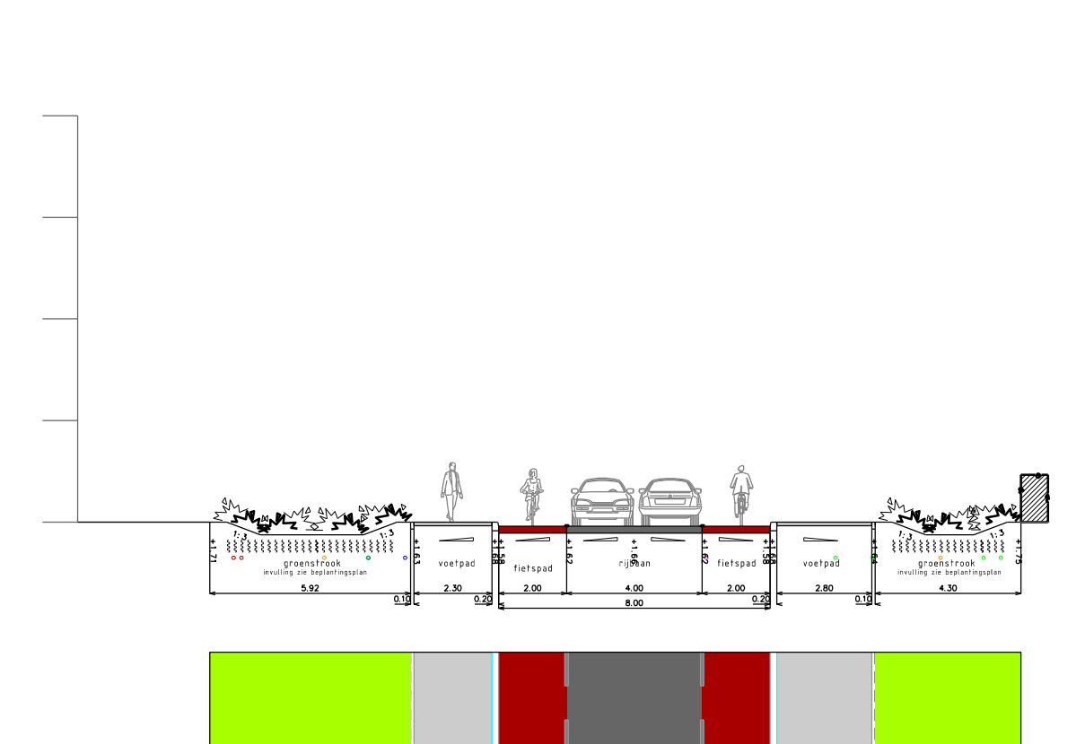
Profiel B-B'
