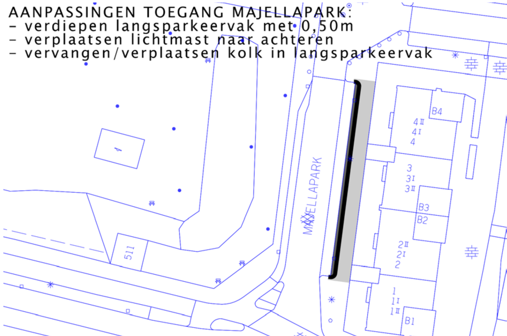
Afbeelding 21: Verruiming bij Majellapark
