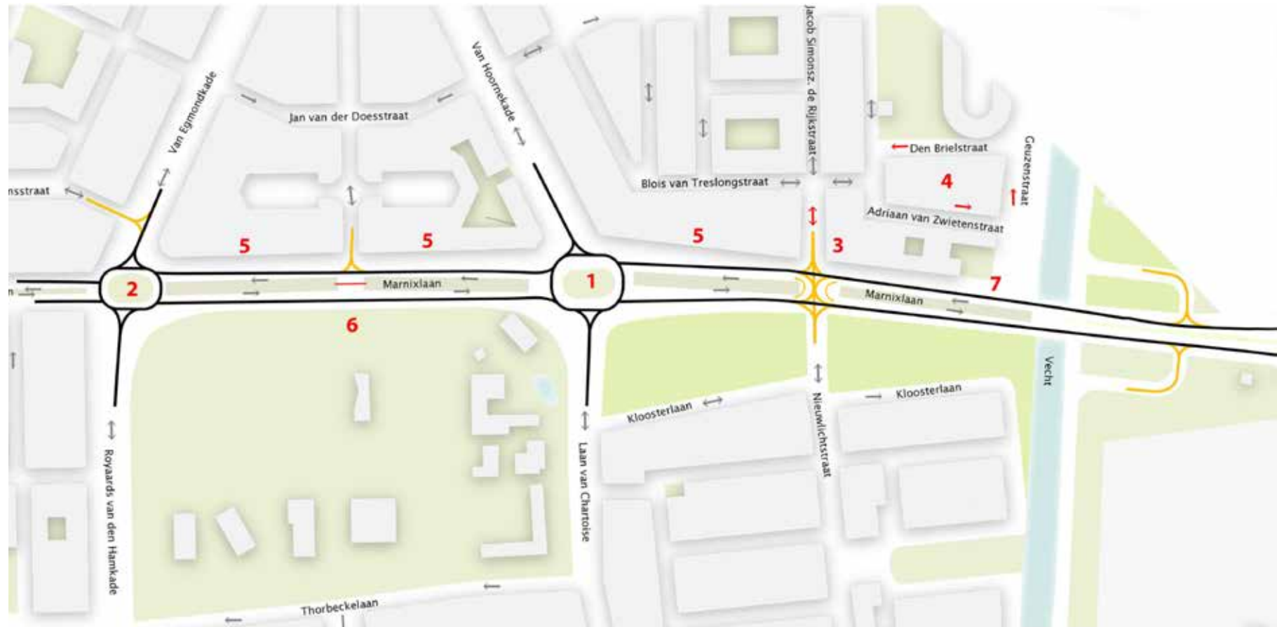
Afbeelding 12: Verkeerscirculatie nieuwe situatie
