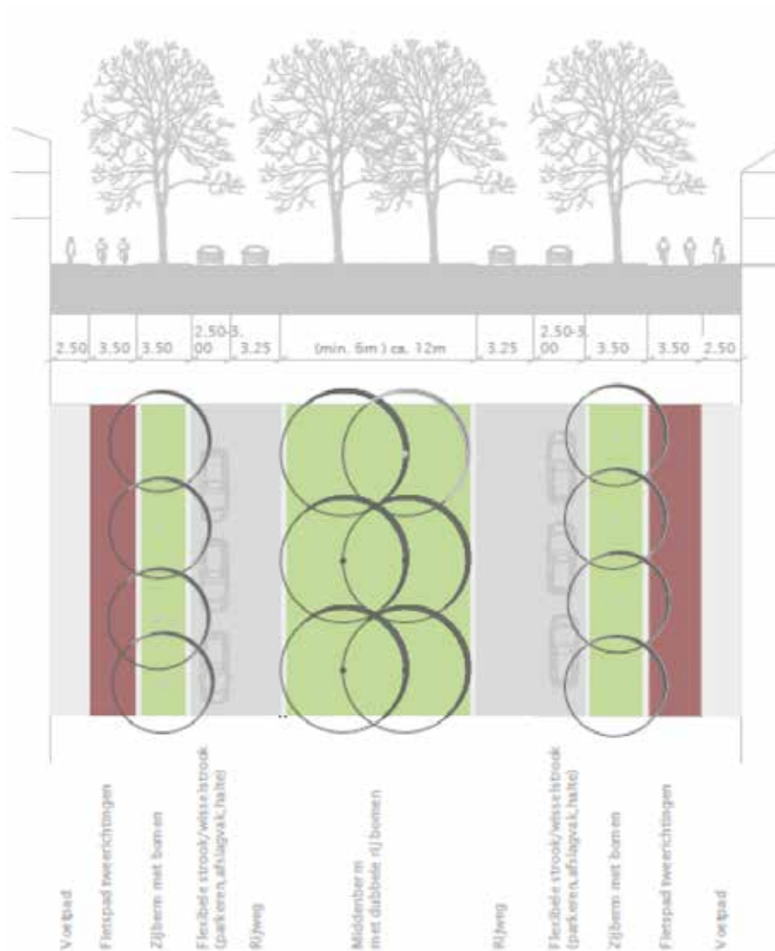
Afbeelding 4, principeprofiel WSB
