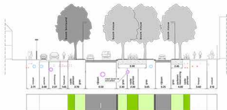
Profiel 15 - Cartesiusweg 2 nabij kruispunt Nijverheidsweg
