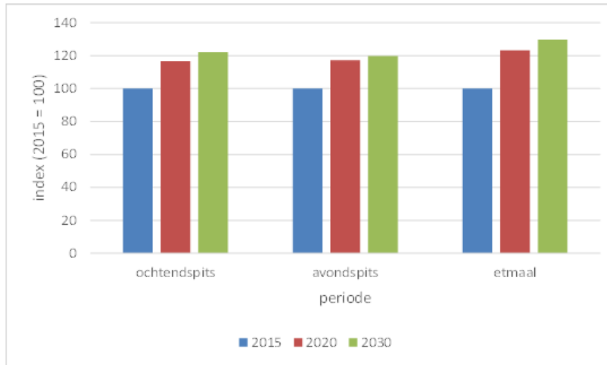
Afbeelding 30: Ontwikkeling auto- intensiteiten WSB-traject, gemiddeld over de wegvakken, bron: projectmodel WSB
