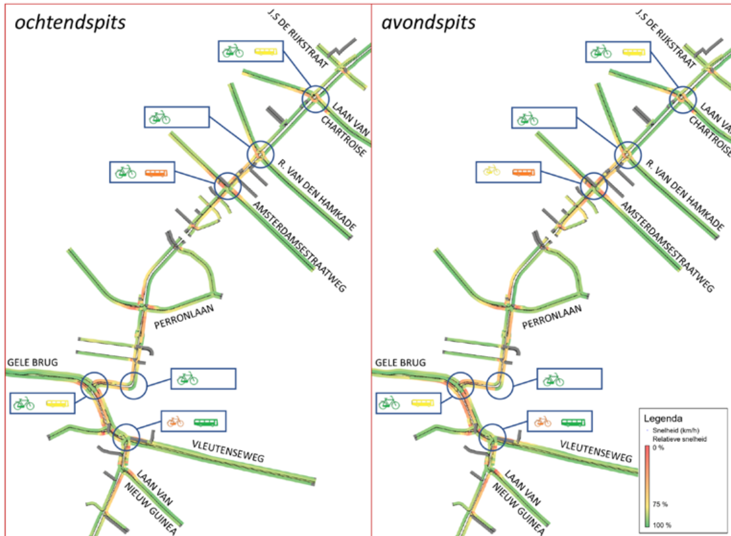
Afbeelding 34: Verkeersafwikkeling op de WSB, noordelijke deel
