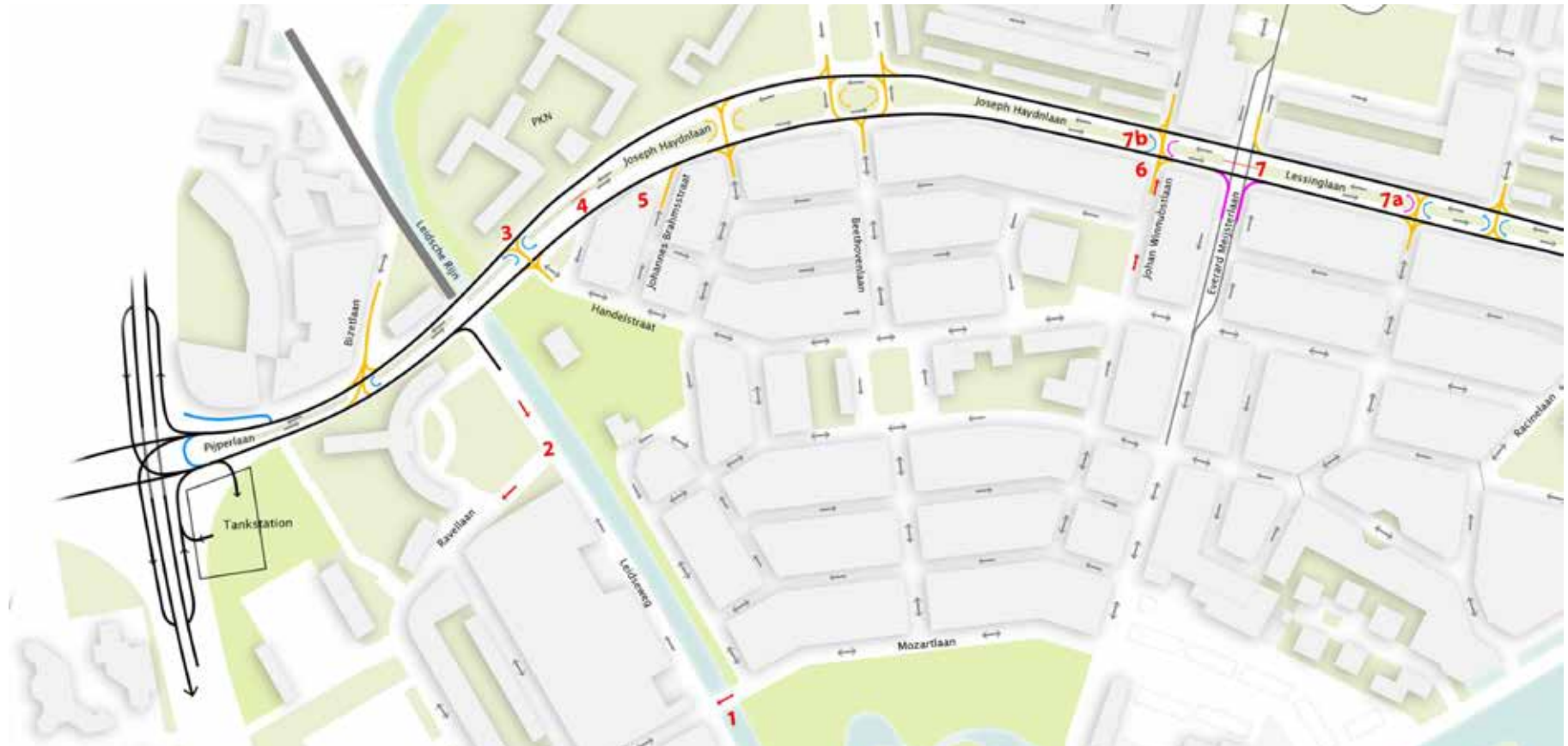
Afbeelding 26: Verkeerscirculatie nieuwe situatie
