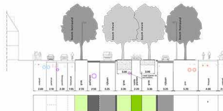
Profiel 16 - Cartesiusweg nabij station Zuren
