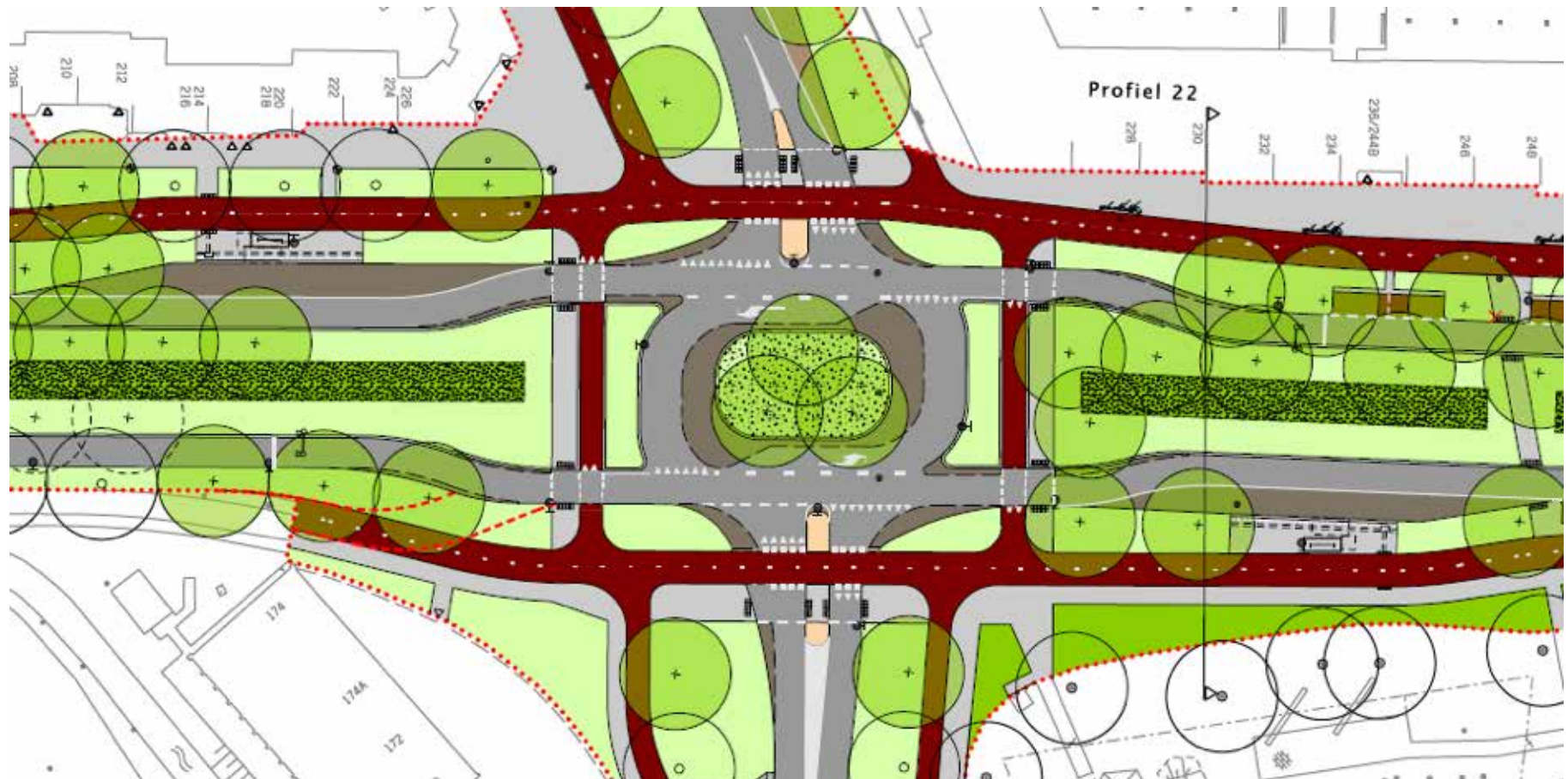
Afbeelding 11: Ontwerp voorrangsp plein Marnixlaan – Van Hoornekade
