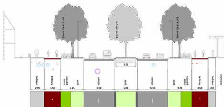
Profiel 14 - Cartesiusweg t.h.v. Schoenerstraat en Fregeatstraat
