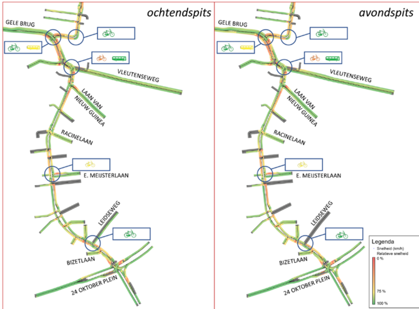
Afbeelding 35: Verkeersafwikkeling op de WSB, zuidelijk deel
